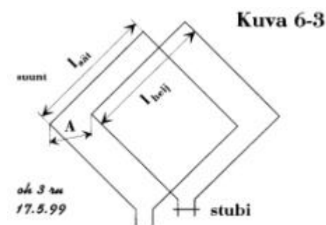
2-elementtinen kvadiantenni
